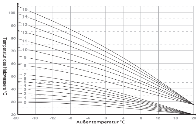
Abb. 27 Diagramm der Heizkurven.
