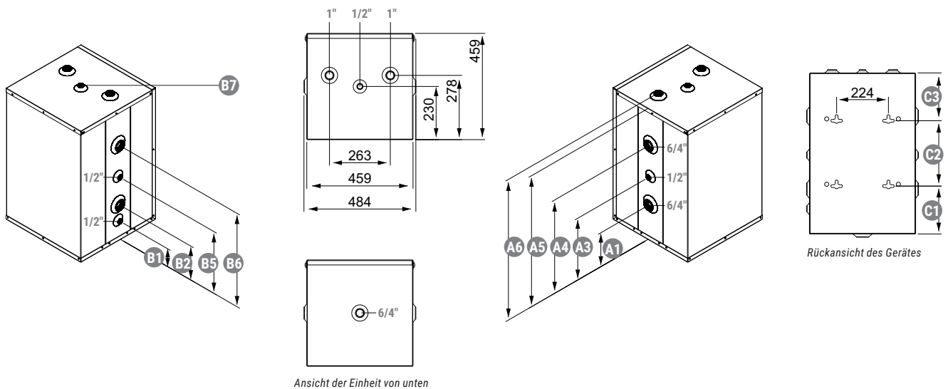
Schema HT BW 40 • 60 L
